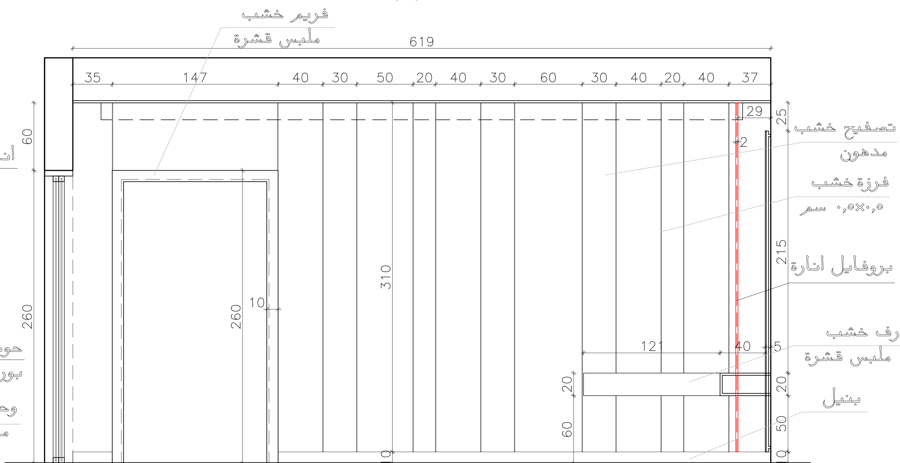
Elevation (D)
