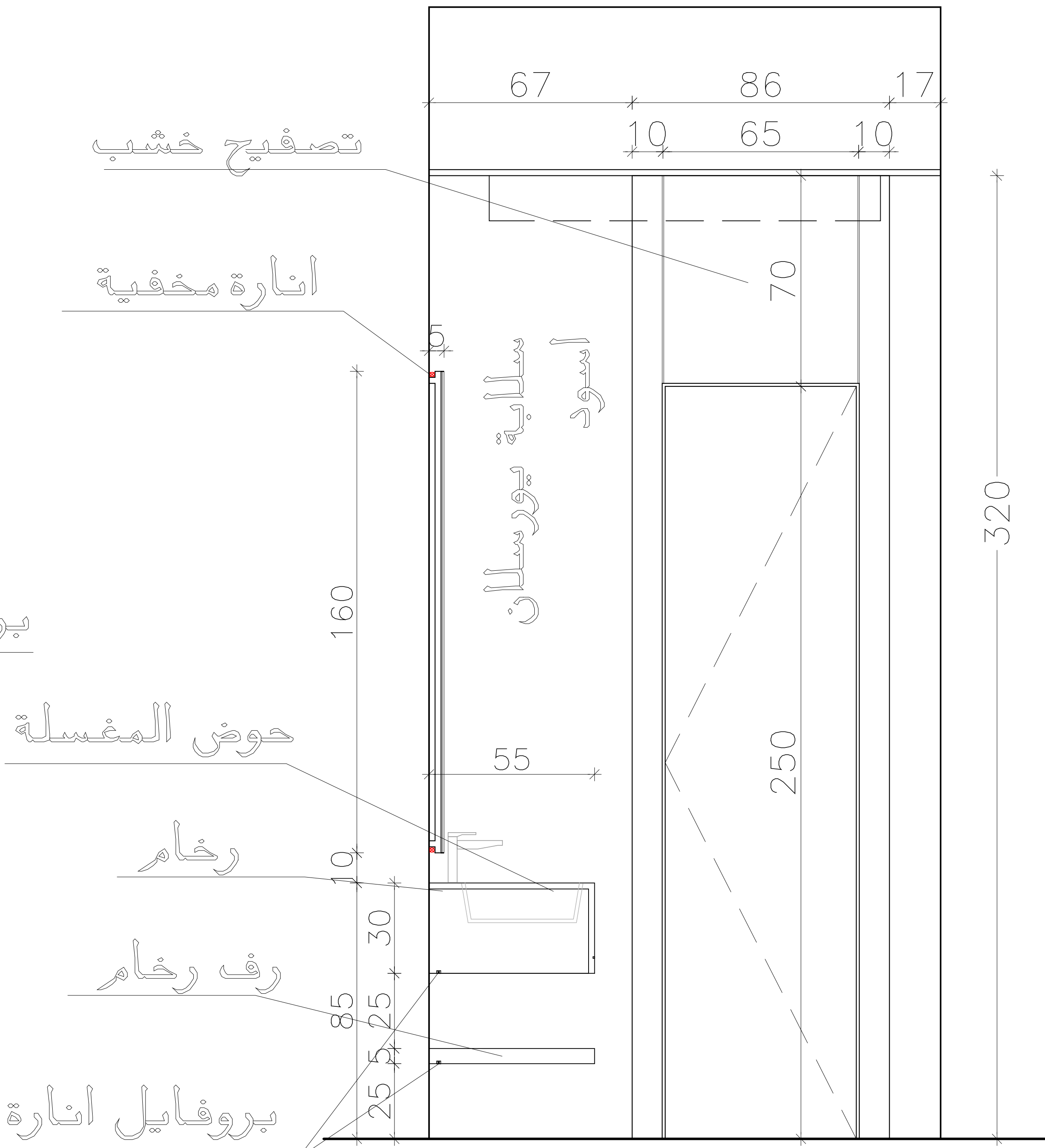
Elevation (D)
