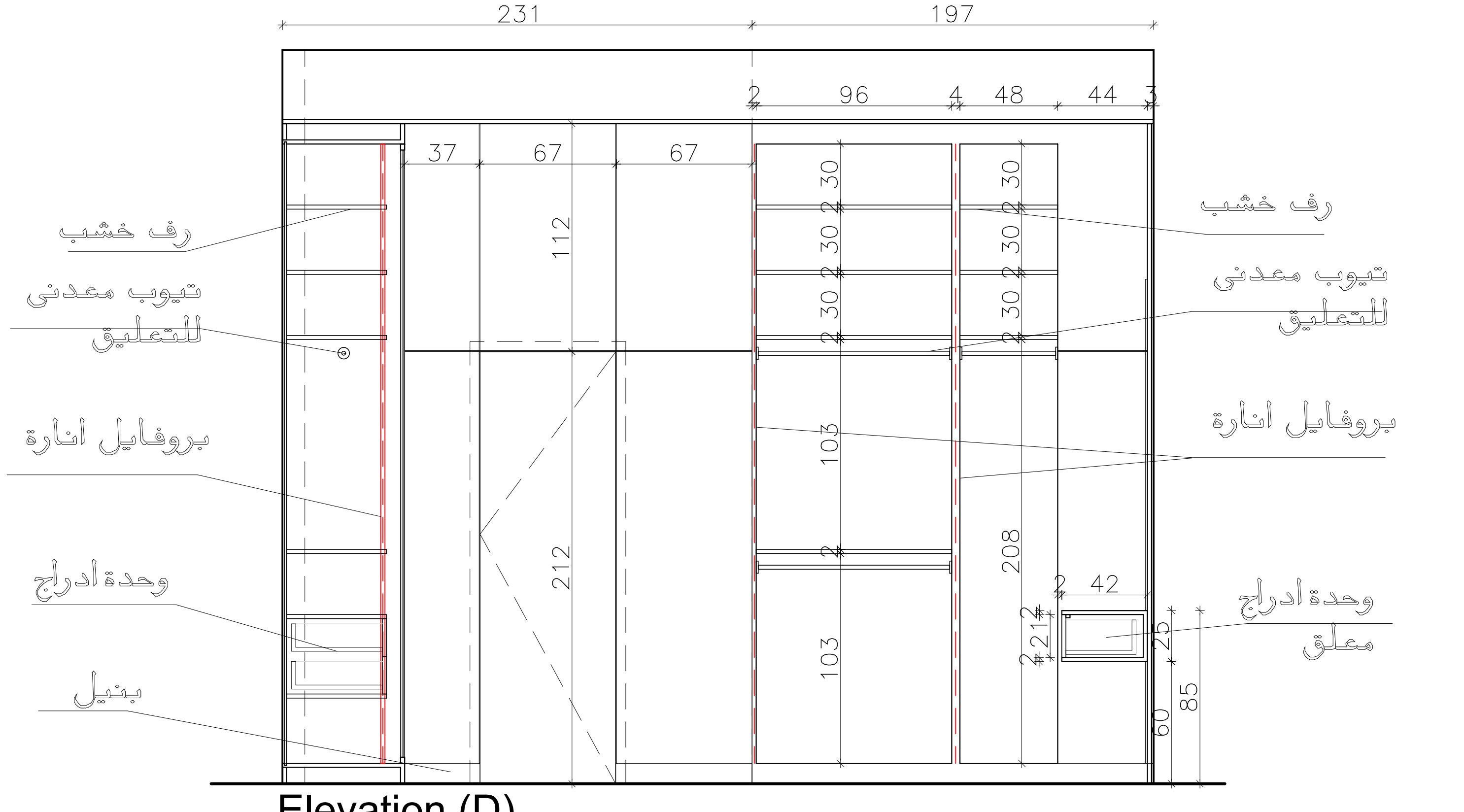
Elevation (D)
