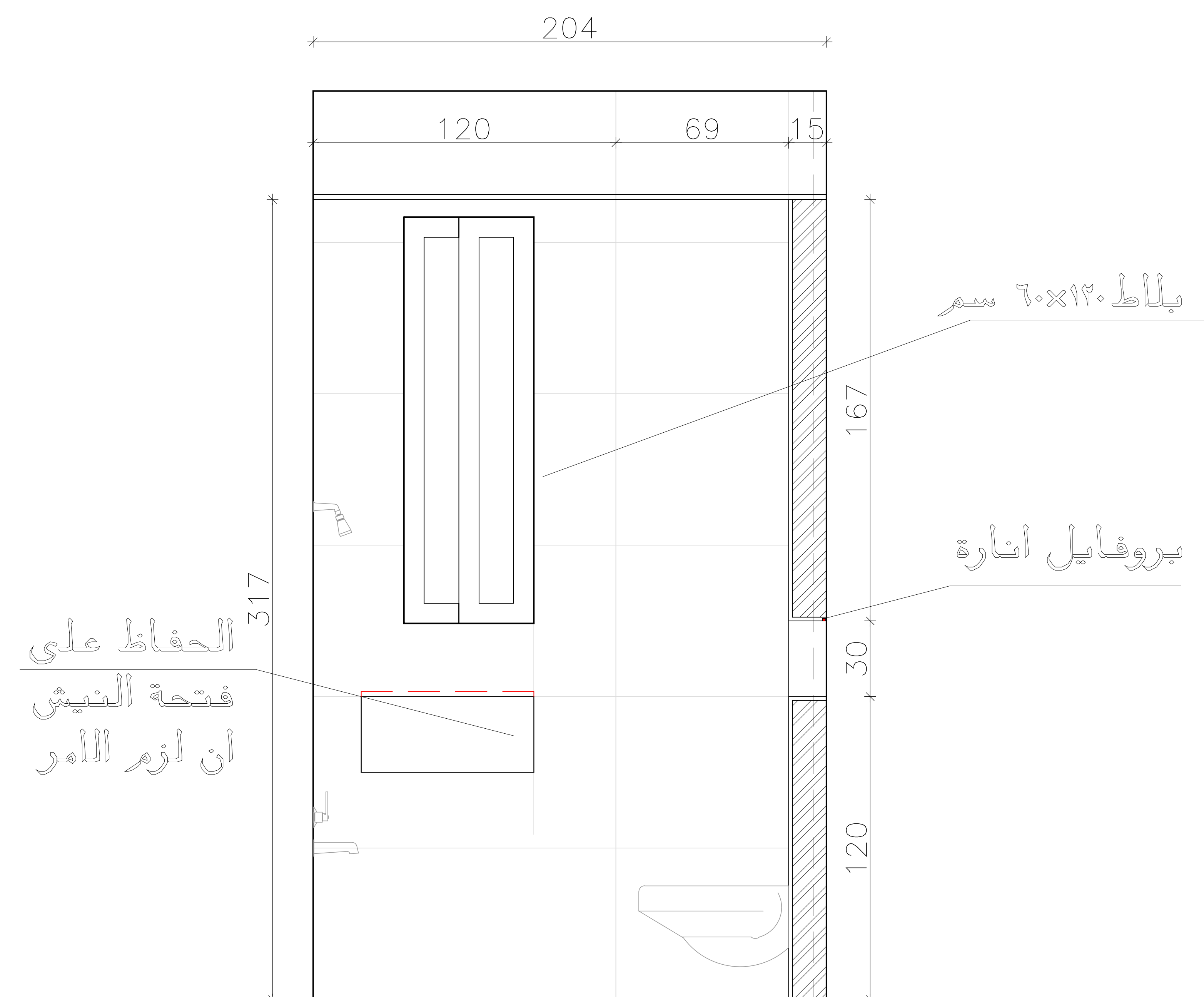
Elevation (D)
