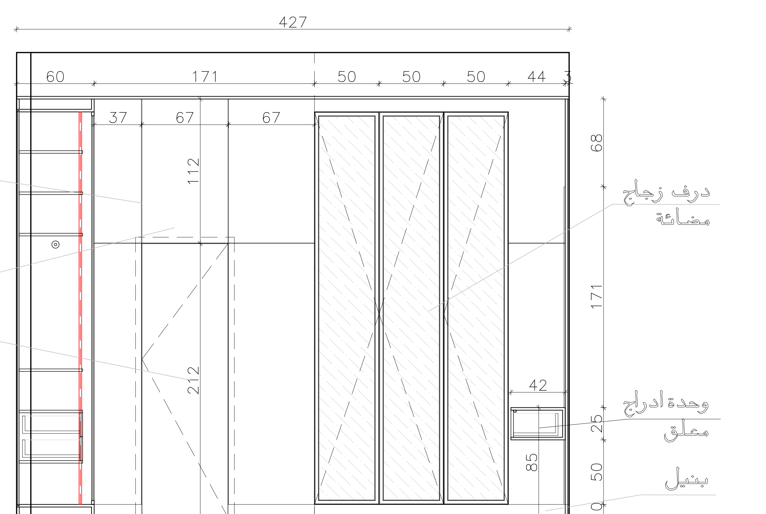
Elevation (D)
