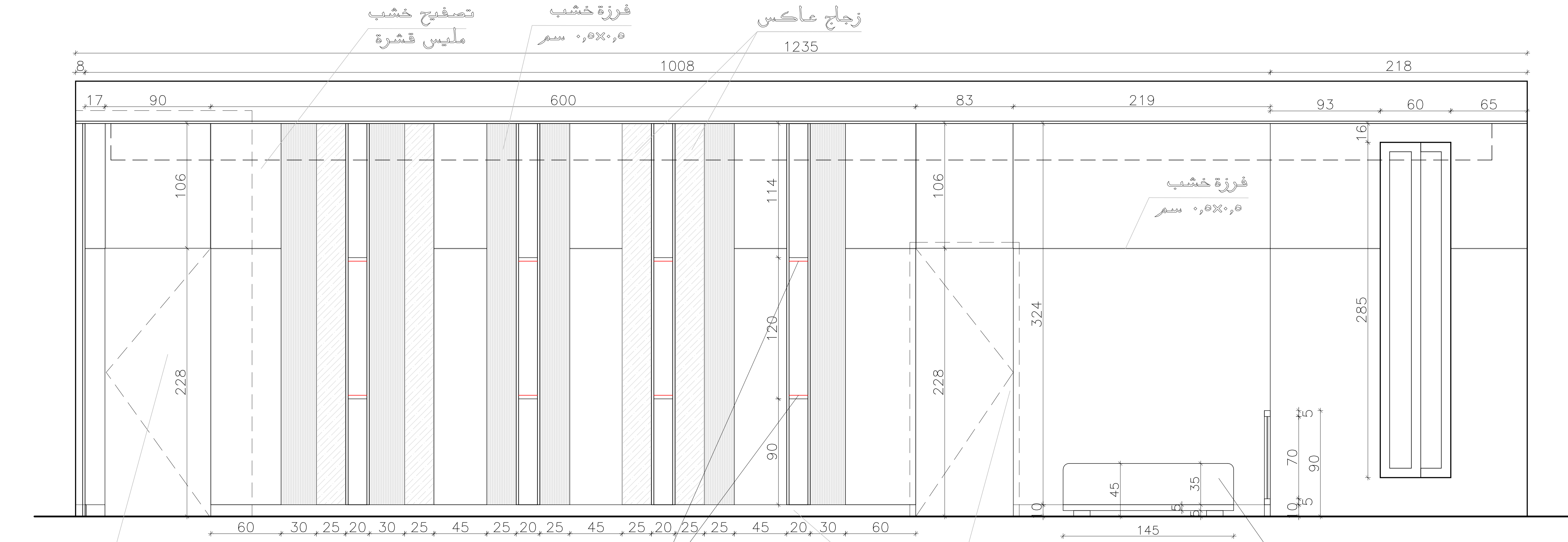
Elevation (D)
