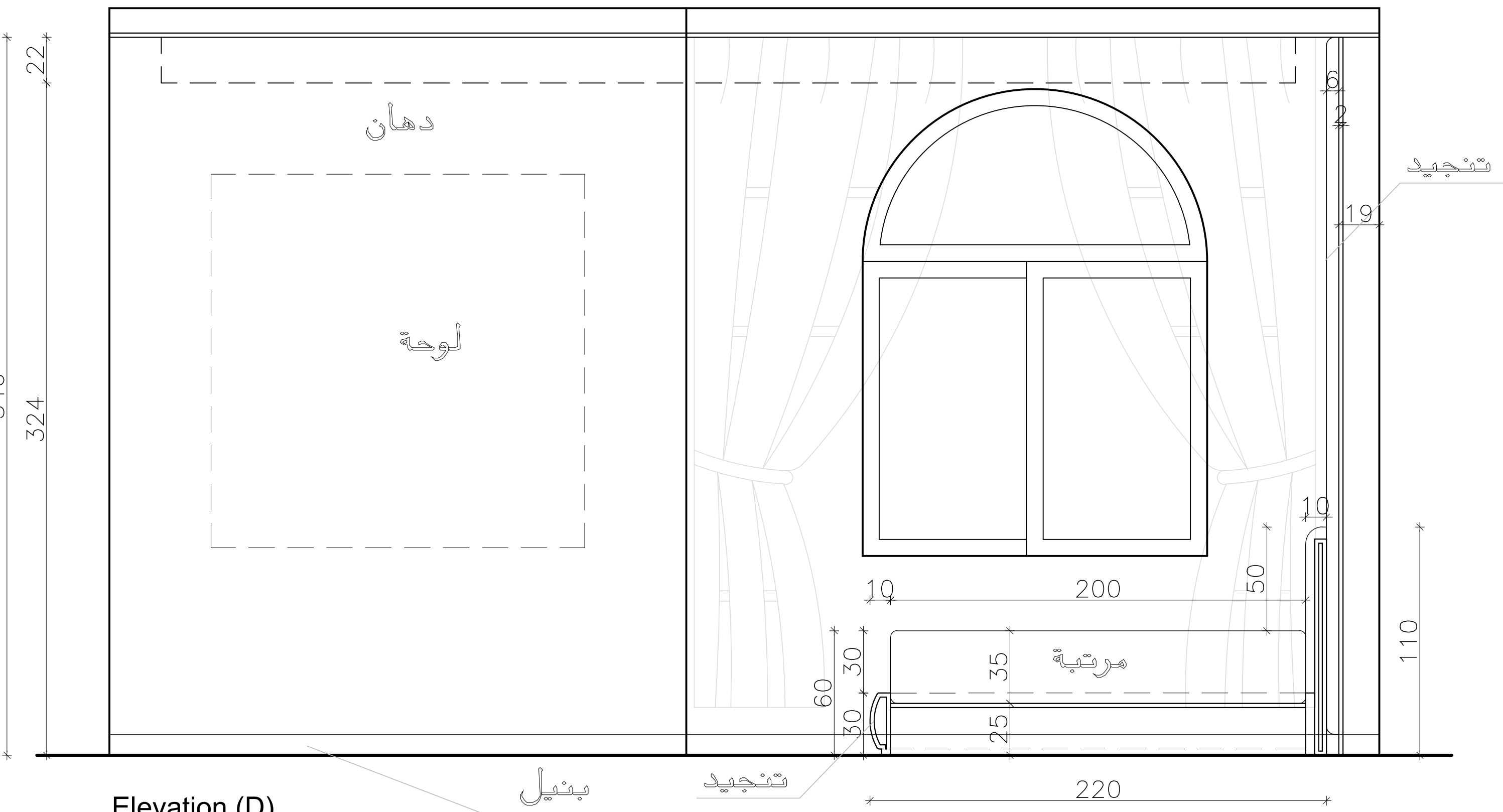
Elevation (D)
