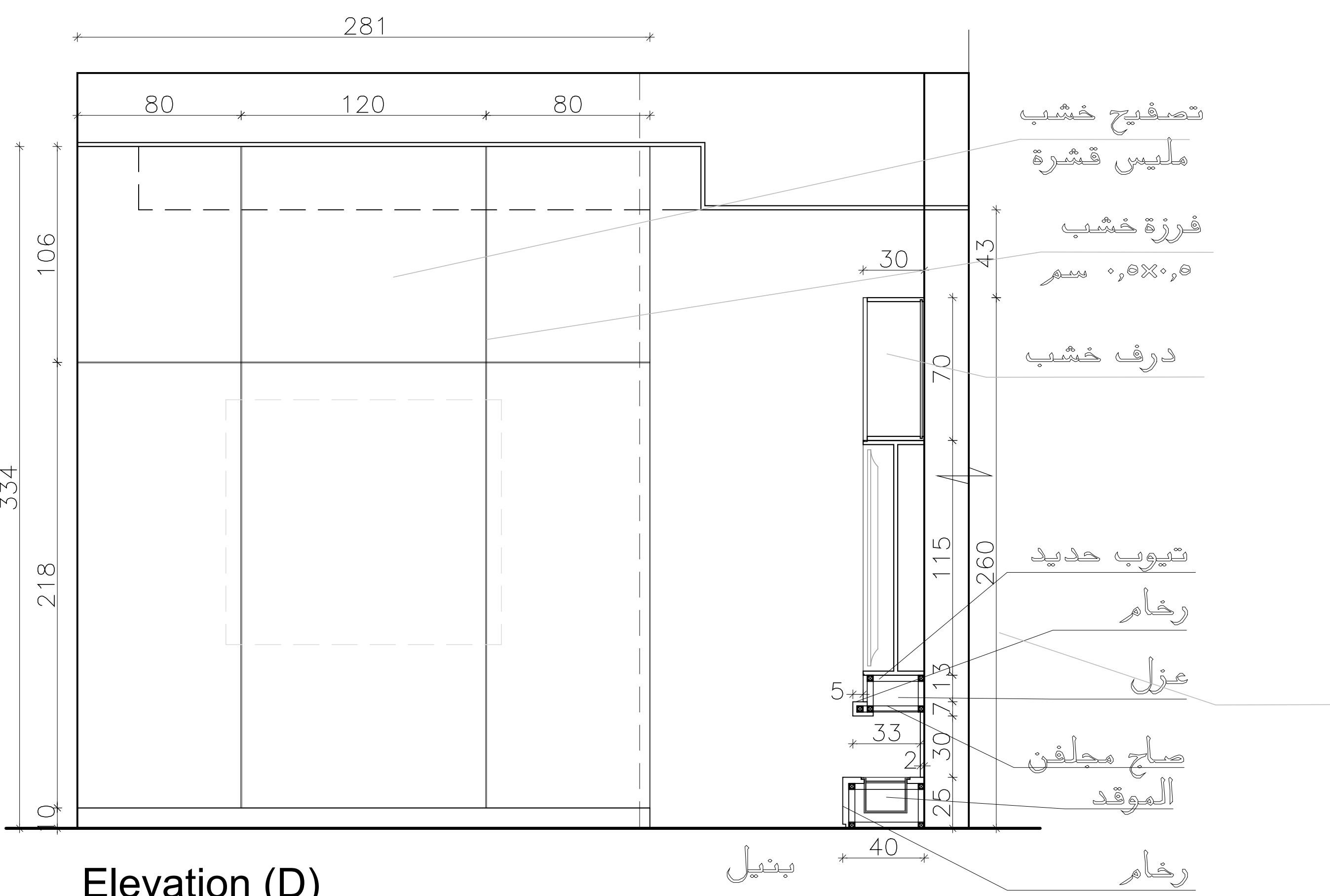
Elevation (D)
